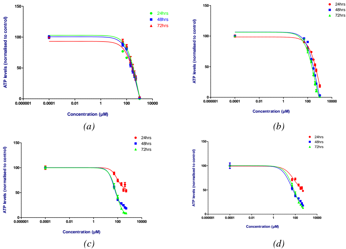
Fig. 3. Cell viability studies of triphenylarsonium derivatives 3 and 4 : (a), Cell Titre Glo assay of zwitterion 3 ; (b) Cell Titre Glo assay of thioacetate salt 4 ; (c), MTT assay of 3 ; (d) MTT assay of 4 .
