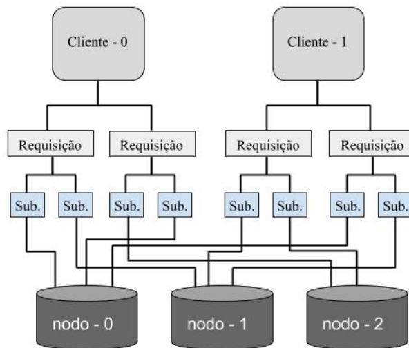
Figura 1. Exemplo básico de funcionamento do simulador.
