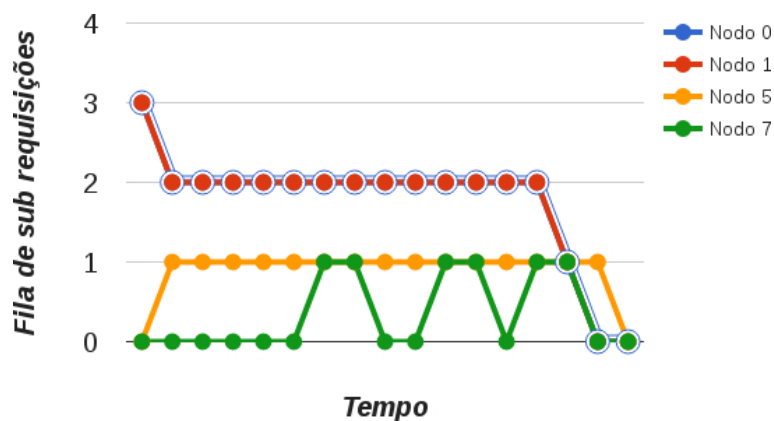
Figura 3. Fila de sub-requisições durante uma execução.
