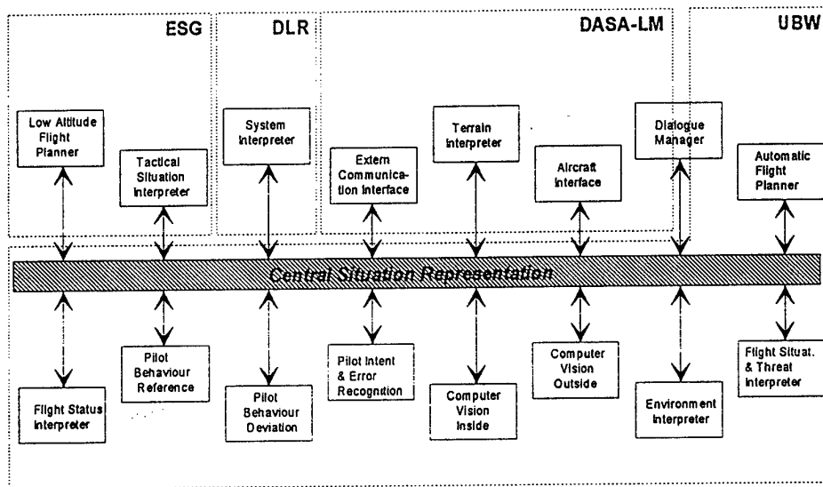
Fig. 2: CAMA Modules
