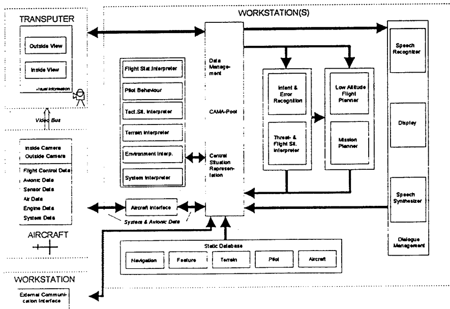
Fig. 2: CAMA Modules
